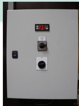
Steuerung der Heizung mit modulierendem Thermostat und 5-stufigem Geschwindigkeitsregler.
